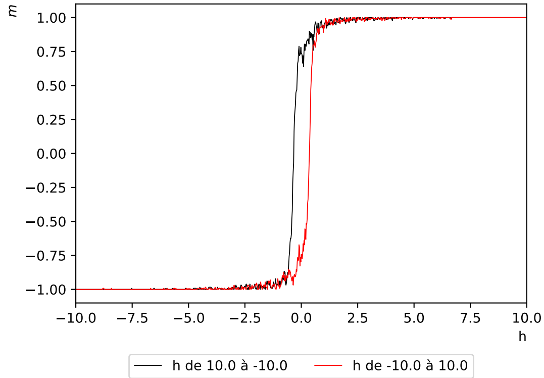
Hystérésis de l'aimantation - réseau de taille L=16 - champ magnétique d'amplitude h=10 à T=2.5
